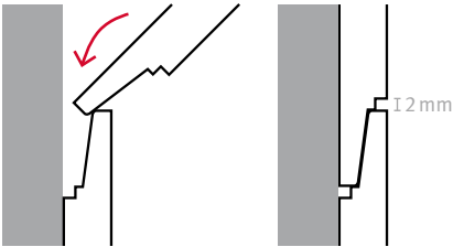
Vertikalsnitt
