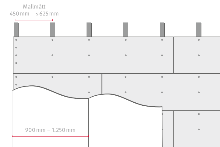
Ändlöst lagda EGGER Ergo Board med gipsskive beläggning med mallmått 450 mm
