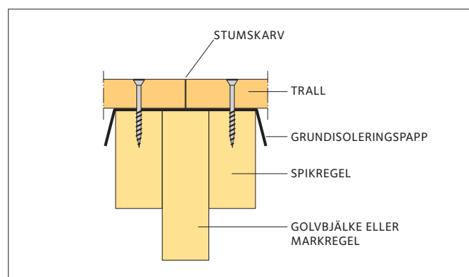
Figur 5 Översidan på underliggande konstruktion bör fuktskyddas med grundisoleringspapp.
