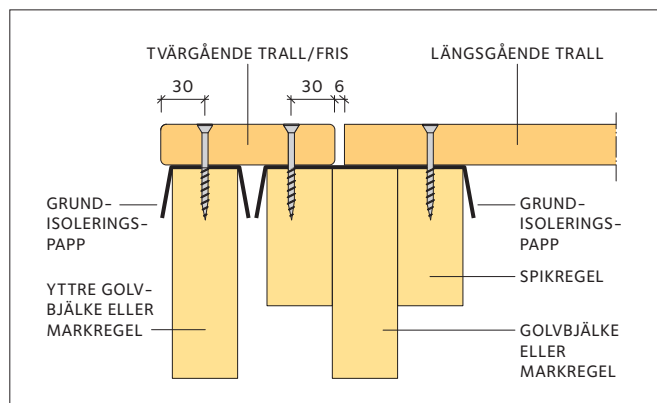
Figur 6 Tvärgående trall, så kallad fris, monterad för att dölja ändträytor på trädäckets kortsidor. Extra stöd genom påsalning av spikreglar innanför den yttre golvbjälken eller markregeln. Trallbrädor ska monteras med 6 mm bred rörelsefog mot fris.
