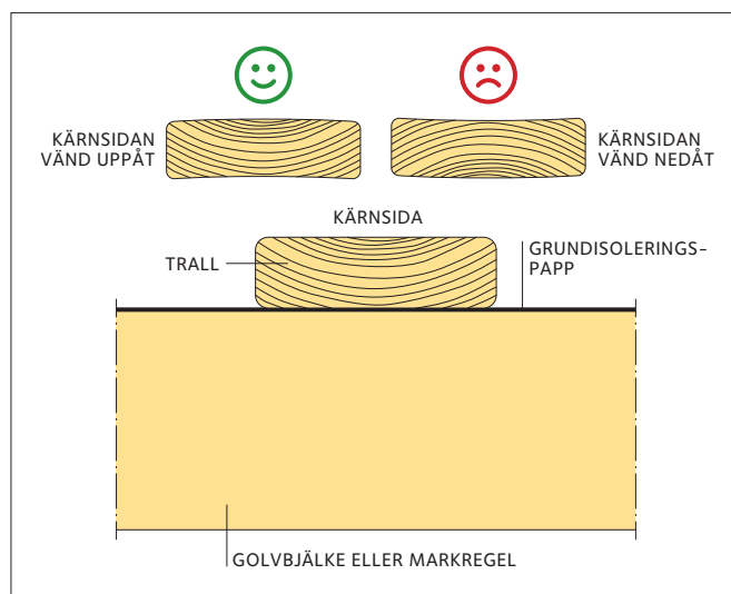
Figur 1 Montera trallbrädan med den bästa sidan vänd uppåt. Om möjligt ska kärnsidan vändas uppåt.
