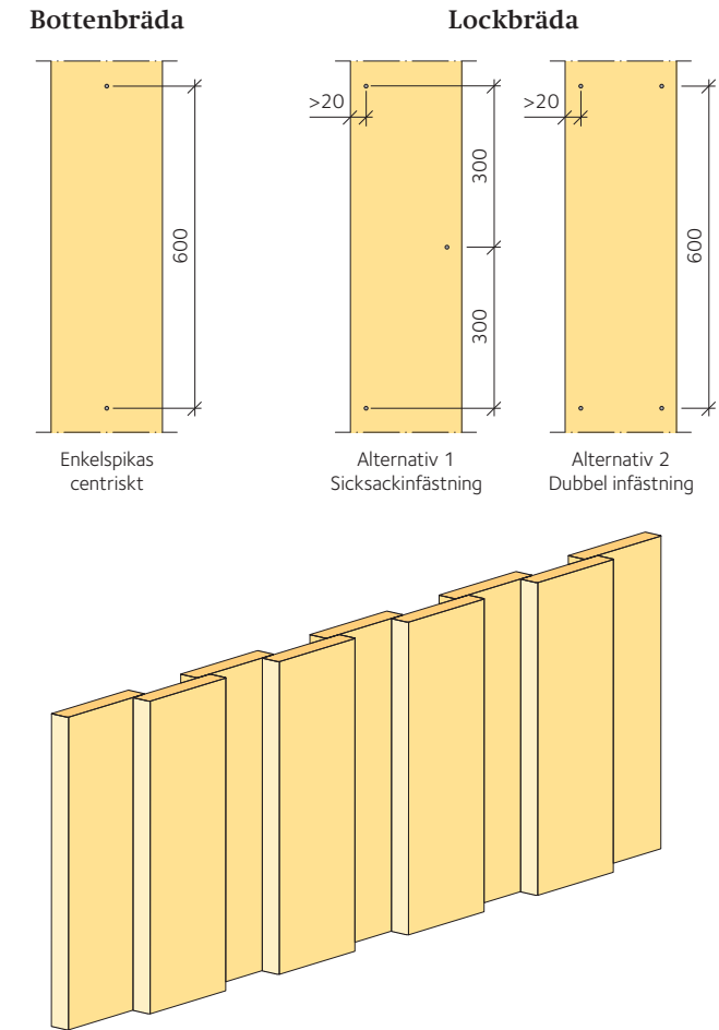
Monterad ytterpanelbräda.
