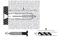
Lättbetong
