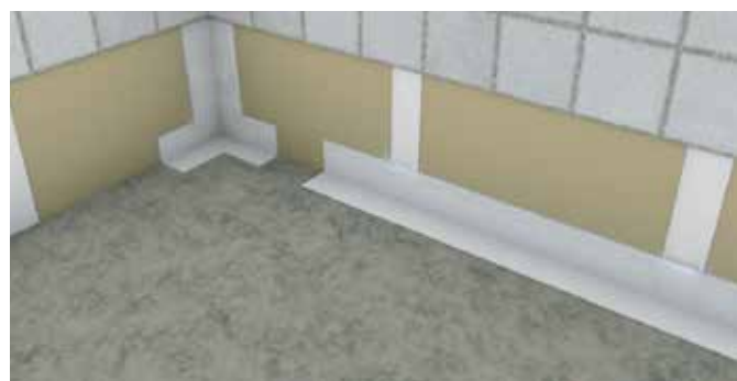
4. Levitä vedeneristettä vedeneristysnauhan alueelle lattian ja seinän liitoskohtaan.
