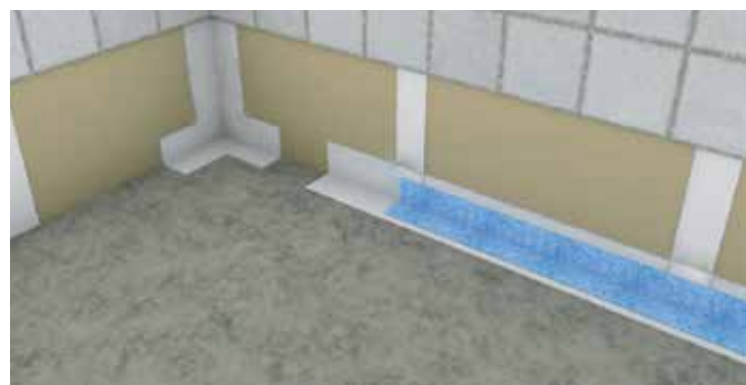
5. Paina nauha kiinni tuoreeseen vedeneristeeseen. Käytä SCHÖNOX iFIX -vedeneristeliimaa, jos kiinnität WetStop KL -nauhaa. Kaikissa tapauksissa tiivistys-/vahviketarvikkeiden tulee limittyä vähintään 5 cm päällekkäin.
