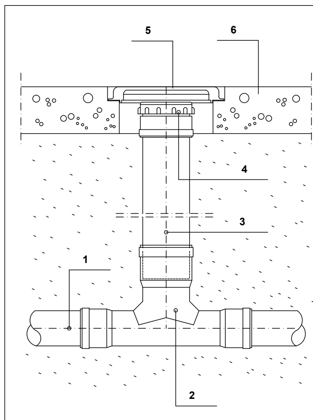
Kuva 84. Esimerkki rakennuksen sisäpuolisesta puhdistusluukusta ja tarkastusputkesta.
