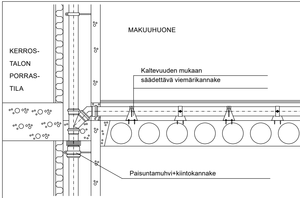
Kuva 42. Vaakaviemärin kannakointi ns. asennuslattiassa.
