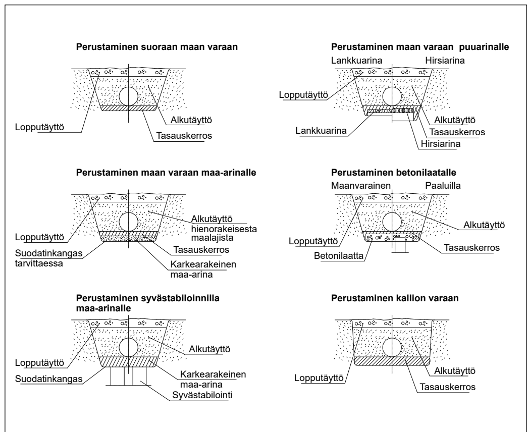
Kuva 45. Putkiarina. Arina voidaan tehdä sinkitystä profiiliteraslevystä, betonista tai sopivasta maa-aineskerroksesta.
