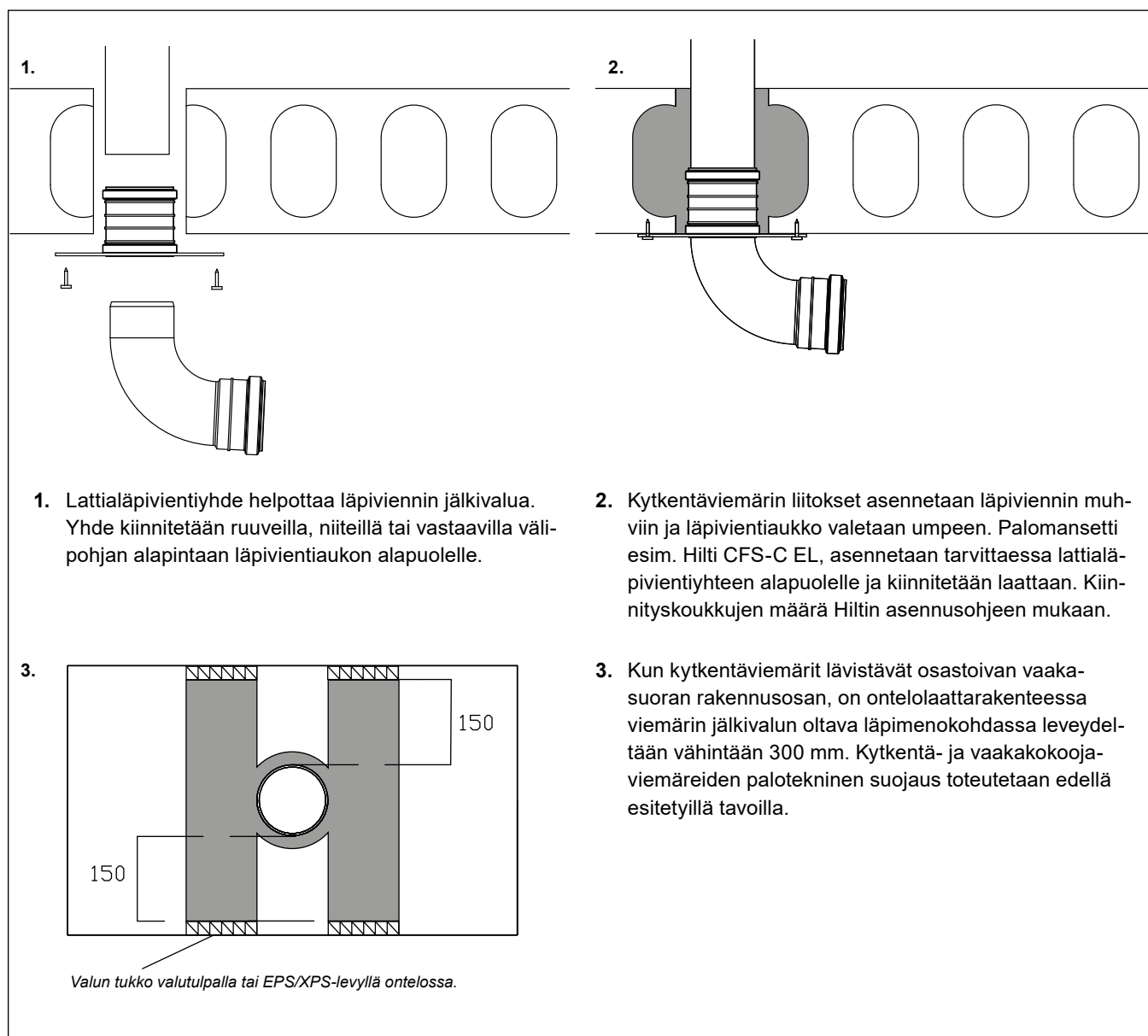
Kuva 34. Lattialäpiviennit.
