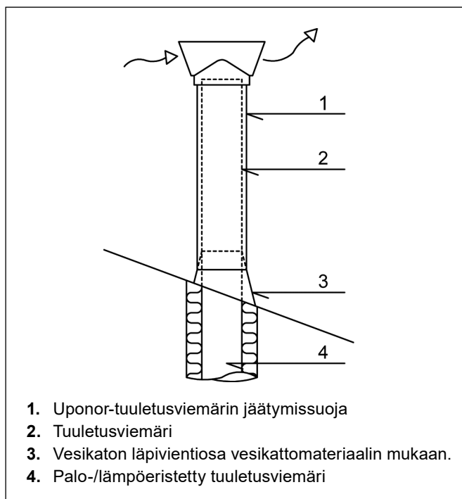
Kuva 83. Uponor-tuuletusviemärin jäätymissuoja asennettuna tuuletusviemärin vesikaton yläpuolisen osan päälle.
