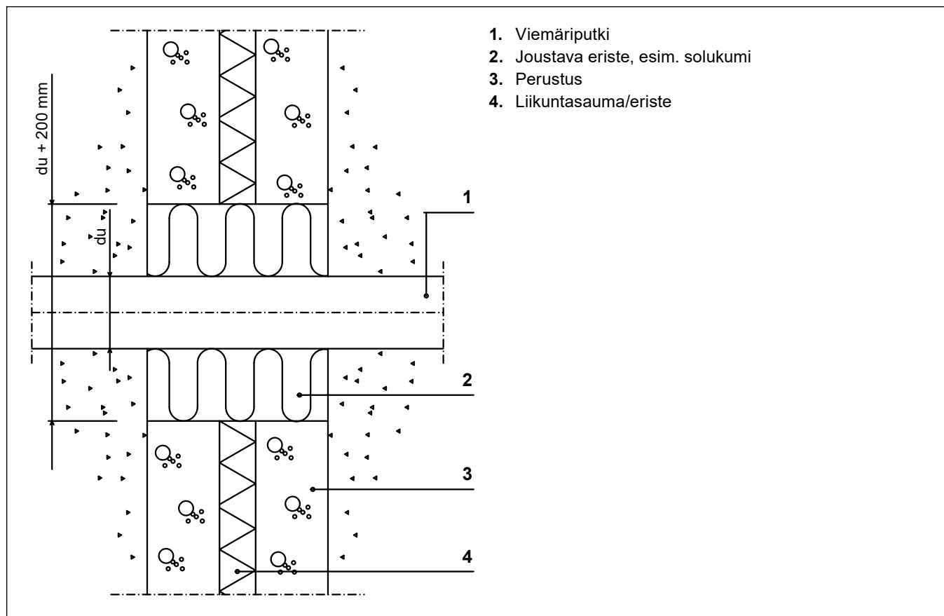
Kuva 47. Maahan asennetun viemäriputken läpivienti liikuntasaumallisen rakenteen läpi, palo-osastoimaton.
