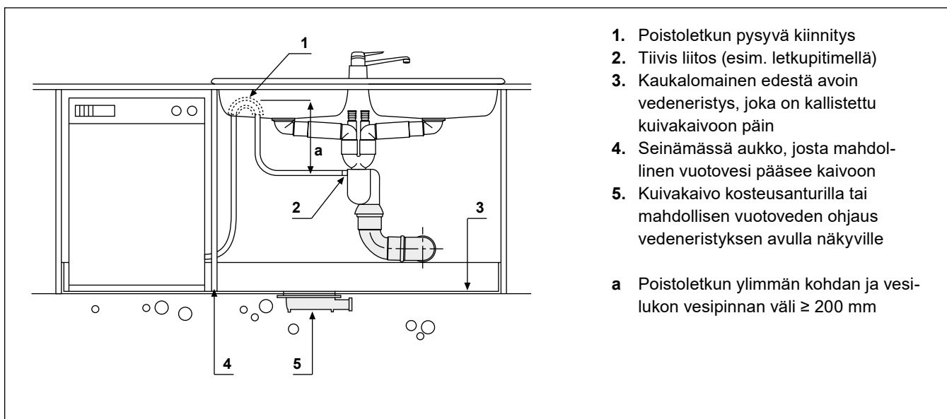
Kuva 70. Astianpesukoneen liittäminen viemäriverkostoon astianpesualtaan vesilukon pesukoneliitännän kautta.
