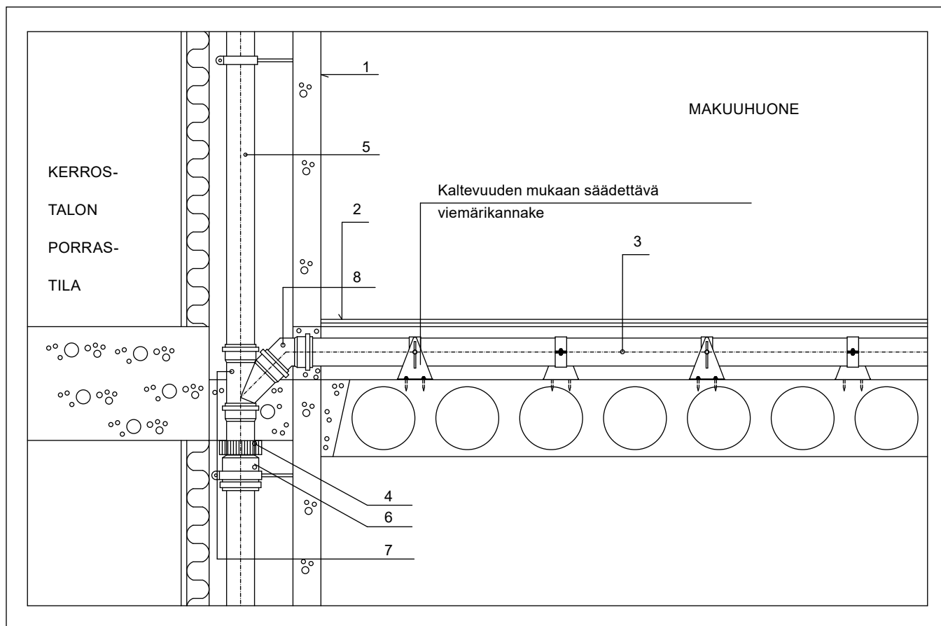
Kuva 21. Esimerkki kytKentä- ja vaakakokoojaviemäriin asennuksesta ns. kerroslattian yhteydessä. Palomansetillä saavutetaan vaadittava palo-osastointiluokka.
