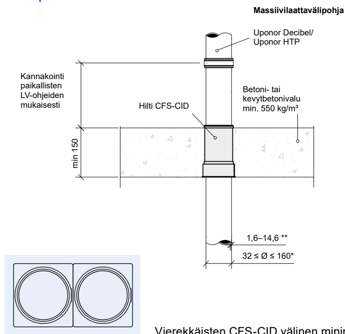
Kuva 28. Palo-osaston läpivienti massiivilaattaväliä pohjassa – palokatkuote Hilti CFS-CID.
