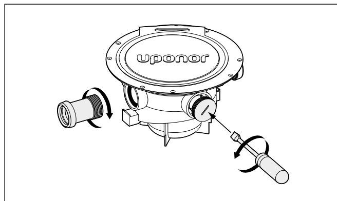
Kuva 73. Sivuliitännän avaaminen.
