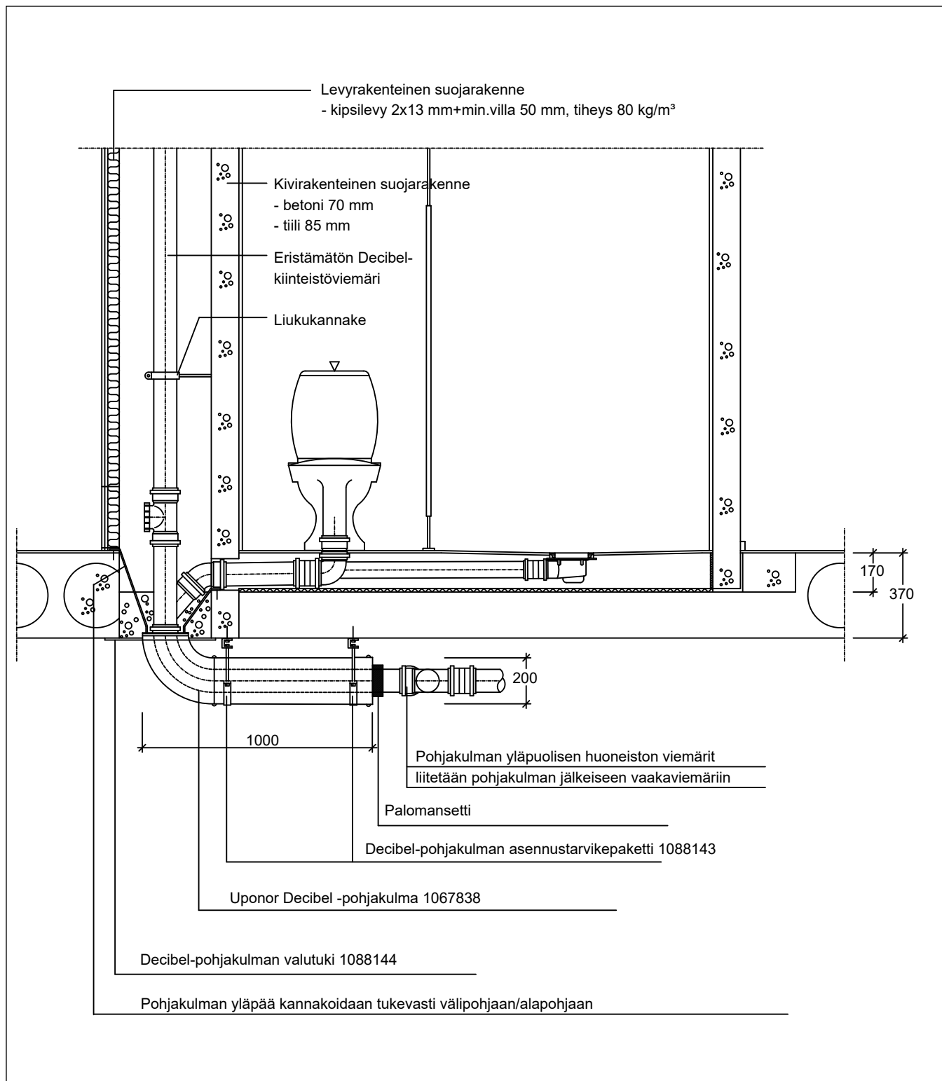
Kuva 22. Eristämättömän Uponor Decibel -kiinteistöviemäriin äänitekniset suojarakenteet, äänitasovaatimus 28 dB(A). Pohjakulman yläpuolista huoneistoa palvelevia viemäriputkia ei liitetä pystykokojaviemäriin, vaan ne johdetaan alapohjan alapuolelle ja liitetään äänenvaimentimen jälkeiseen vaakaviemäriin.
