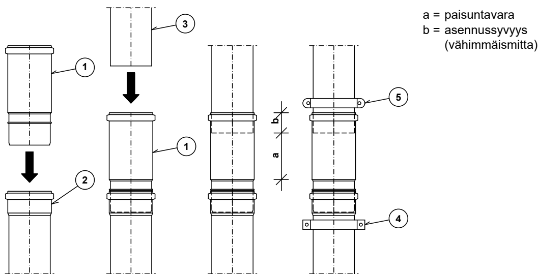
Kuva 40. Uponor Decibel- ja HTP -viemärin paisuntayhteen asennus.
