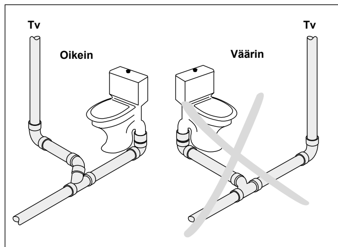
Kuva 66. Tuuletusviemärin liittäminen vaakakokoajaviemäriin.
