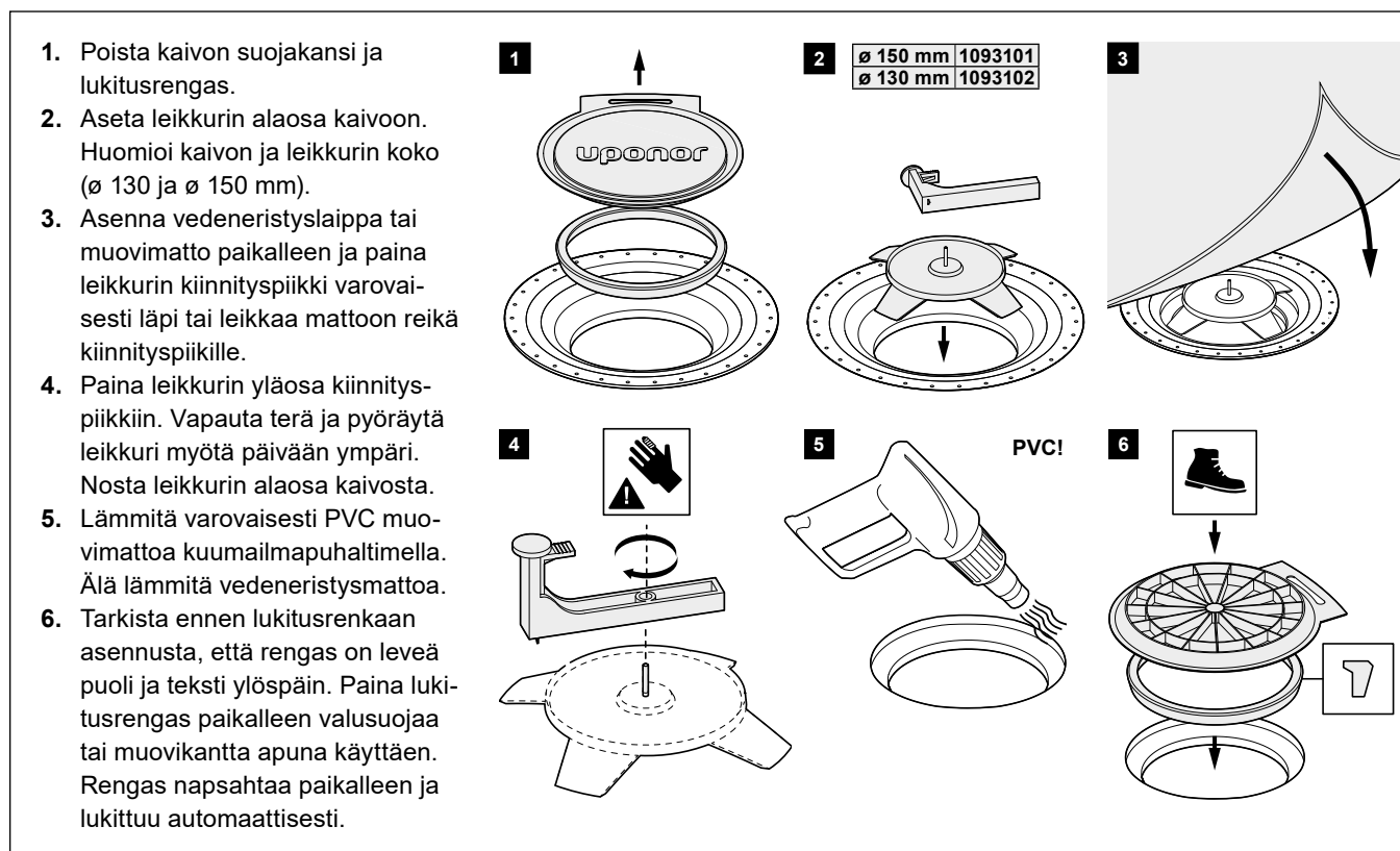
Kuva 80. Leikkurin käyttö ja lukitusrenkaan asennus.
