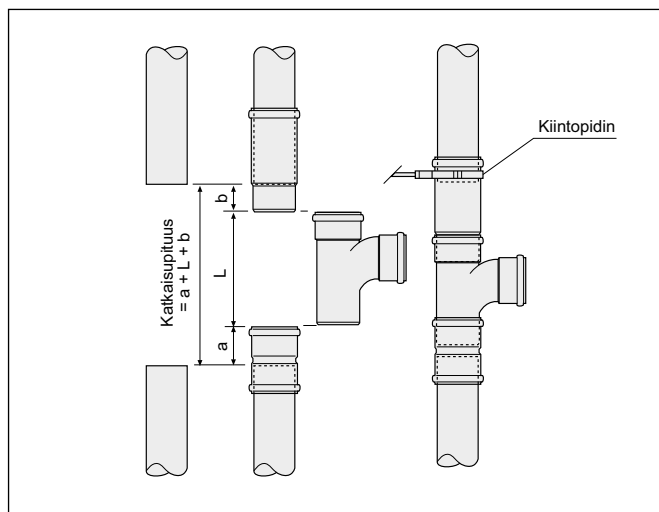
Kuva 51. Haaroitus haarayhteen, kaksoismuhvin ja liitos-/paisuntayhteen avulla.
