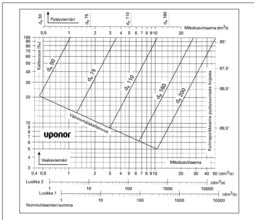
Kuva 37. Uponor-kokoojaviemärin mitoitusdiagrammi.
