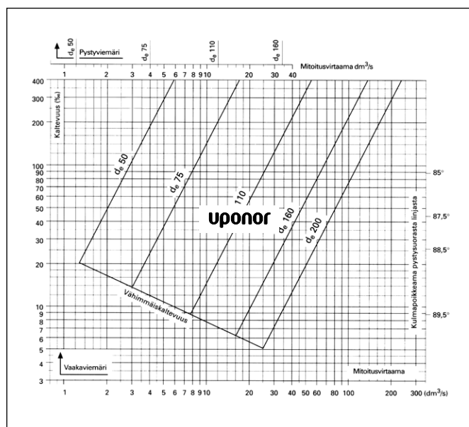
Kuva 39. Mitoitusdiagrammi Uponor-sadevesiviemäriä varten.
