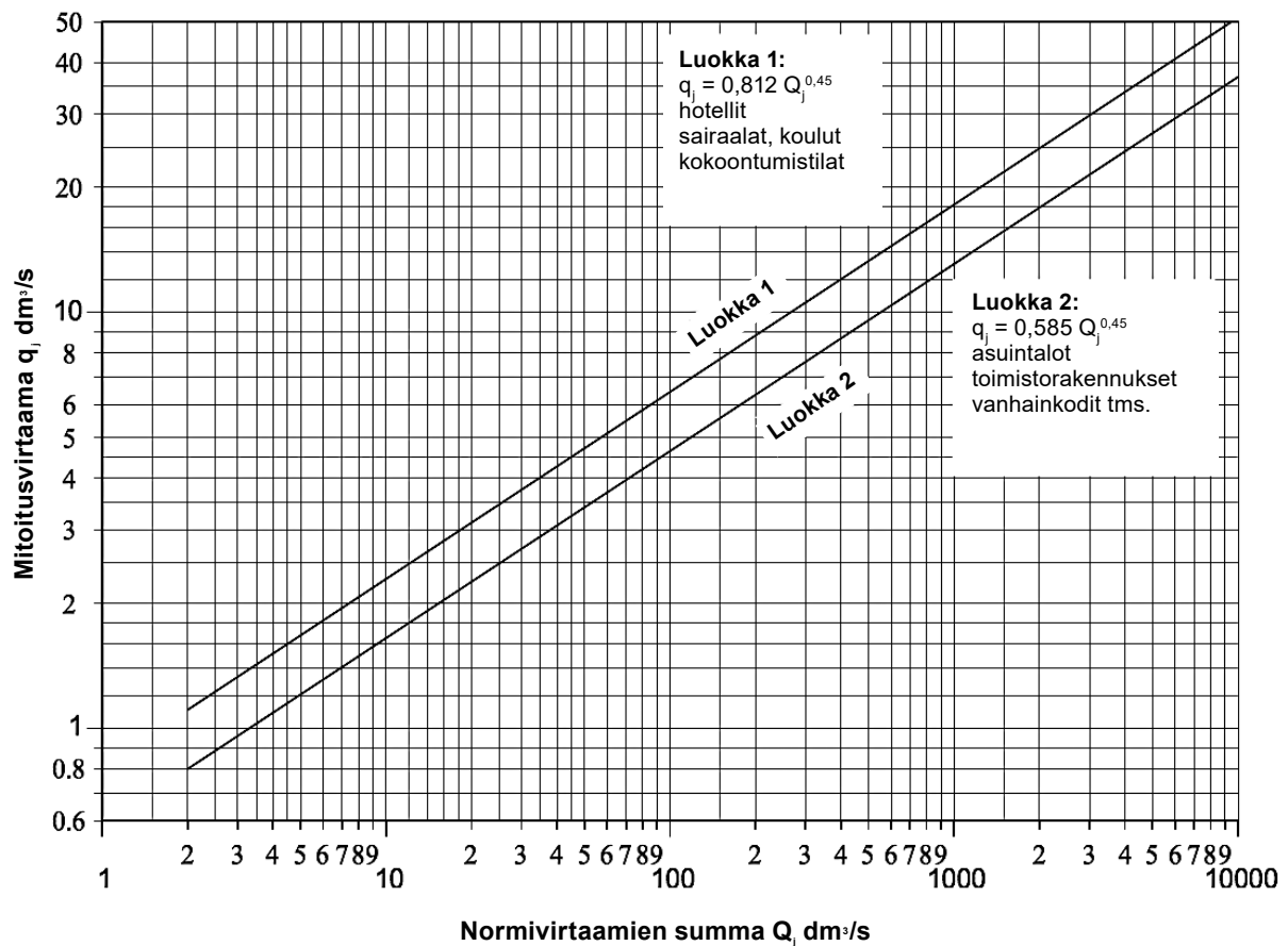
Taulukko 14. Viemärin mitoitusvirtaaman riippuvuus normivirtaamien summasta.
