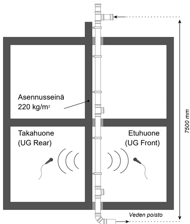
Kuva 3. EN 14366 testausjärjestely (Fraunhofer Institute)
