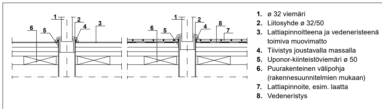
Kuva 68. Esimerkki kytkentäviemärin läpiviennistä kostean tilan puurakenteisessa välipohjassa.
