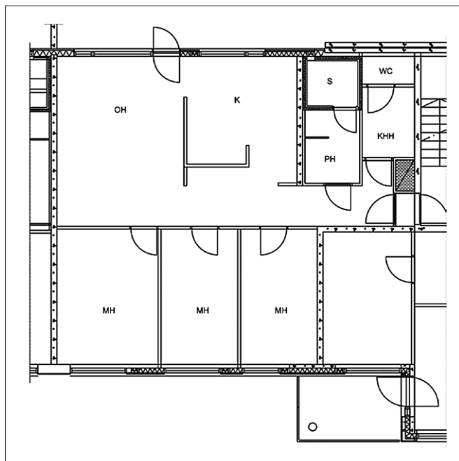
Kuva 8. Hormitila sijoitetaan mahdollisimman etäälle äänitasovaatimuksiltaan vaativista tiloista.
