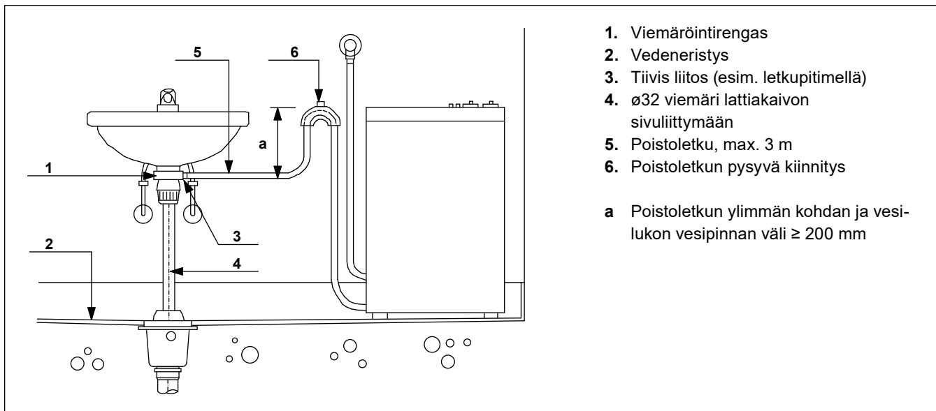
Kuva 69. Pesukoneen liittäminen viemäriverkostoon pesualtaan vesilukon yhteyteen asennetulla viemäröintirenkaalla.
