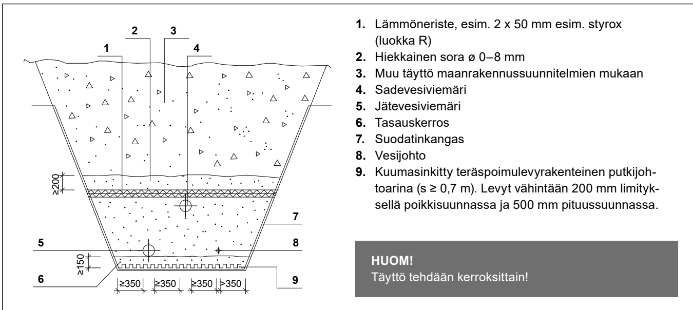
Kuva 45. Putkiarina. Arina voidaan tehdä sinkitystä profiiliteraslevystä, betonista tai sopivasta maa-aineskerroksesta.
