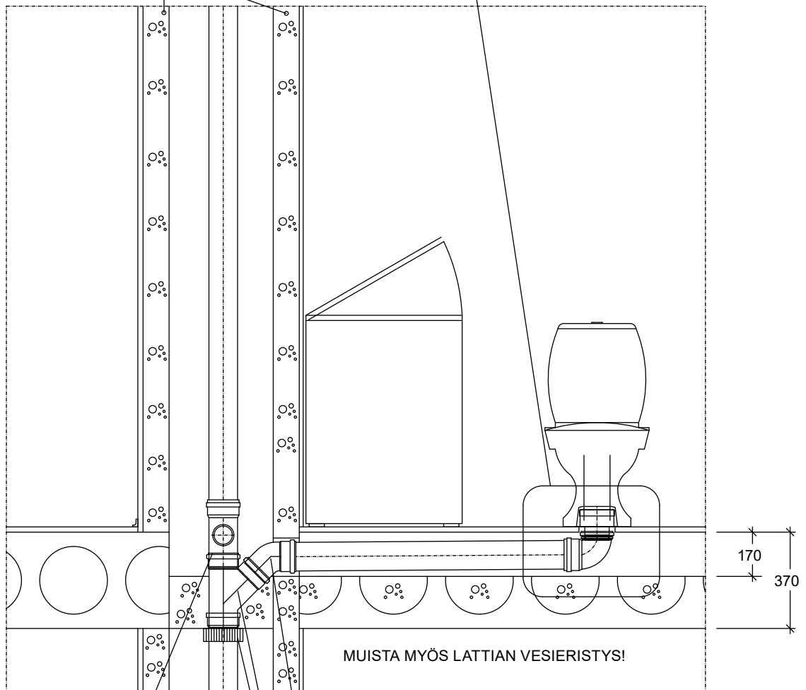
Uponor-haarayhde 110/75-45° nro 1053729
