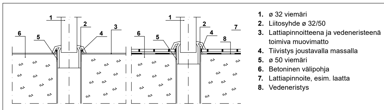
Kuva 67. Esimerkki kytkentäviemärin läpiviennistä kostean tilan betonirakenteisessa välipohjassa.
