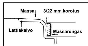
Kuva 79. Drain-massarengas soveltuu massa/harts/epoksilattioille.
