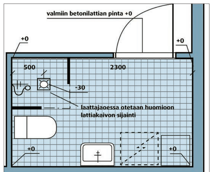
Kuvassa esimerkki märkätilan lattian korkeusasemien merkitsemisestä suunnitelmapiirrookseen.
