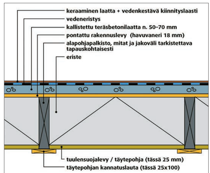
Kuvassa esimerkki märkätilan lattian rakenteesta puurunkoisessa välipohjarakenteessa.
