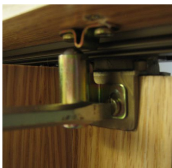
6. Työnnä ovi nippuun ja kiinnitä jarrulevy (F) peitelistaan ruuveilla (e). Säädä kuulalukon korkeus sopivaksi.
