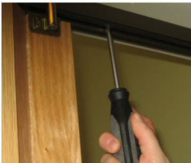
3. Nosta ovi aukkoon ja kiinnitä liukukisko ruuveilla (a) ja peitelistat (C) ruuveilla (b).
