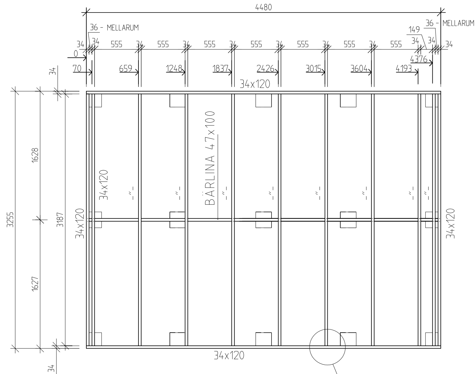
BJÄKLAGSPLAN
