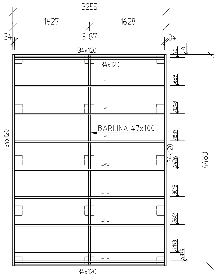
BJÄKLINGSPLAN
