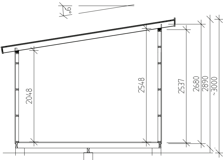
SEKTION A-A
