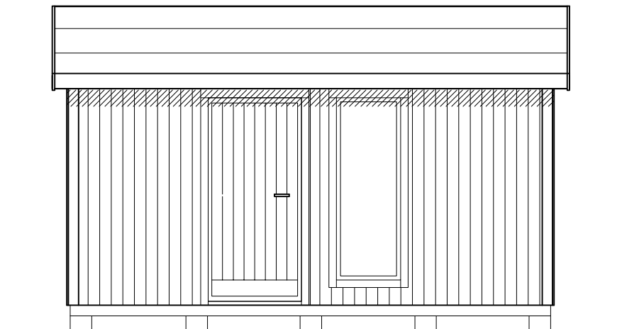
FASAD LÅNGSIDA 1
