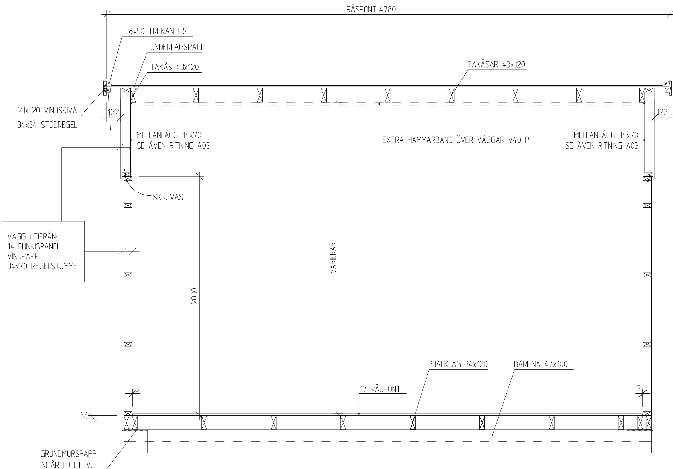
LÄNGDSEKTION
