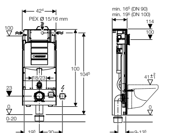
GIS-WC-elementti, edestä käytettävä, h = 112 cm, Tuotenro 461.307.00.5
