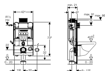
GIS-WC-elementti, päältä/edestä käytettävä, h = 82 cm, tuotenro 461.240.00.1
