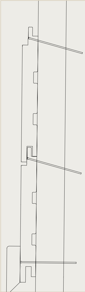
Esimerkki piilokiinnityksestä
