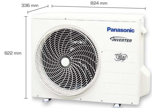
Ulkoyksikkö
