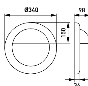
AVL41 häikäisysuojarengas
