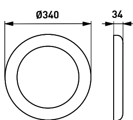
AVL40 koristerengas
