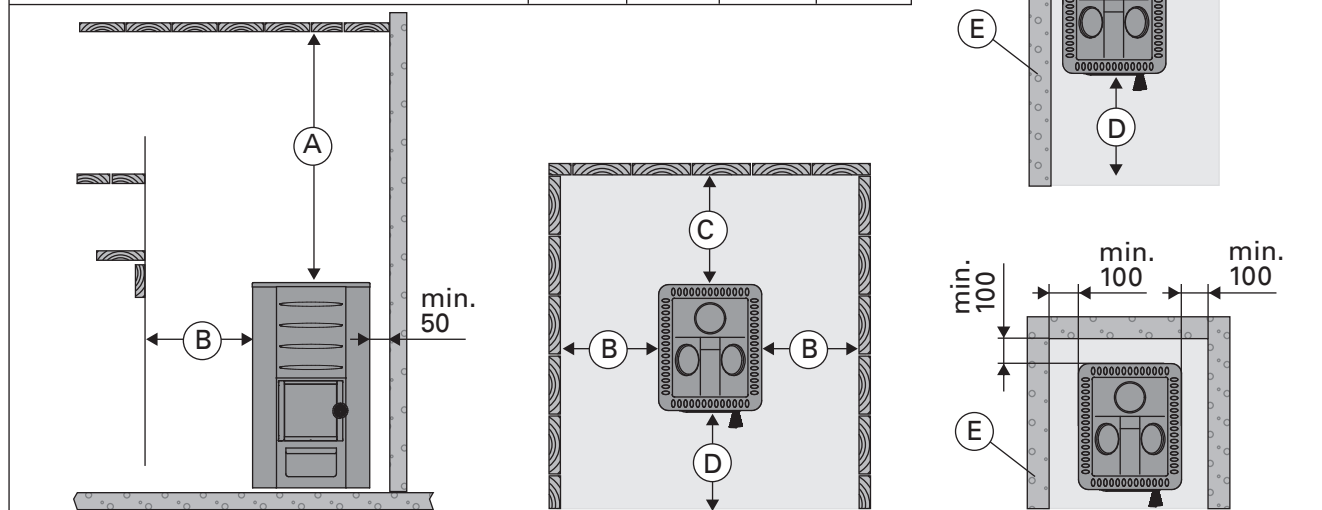
Рисунок 7. Безопасные расстояния (все размеры приведены в миллиметрах) Joonis 7. Ohutuskaugused (kõik mõõtmised millimeetrites)
