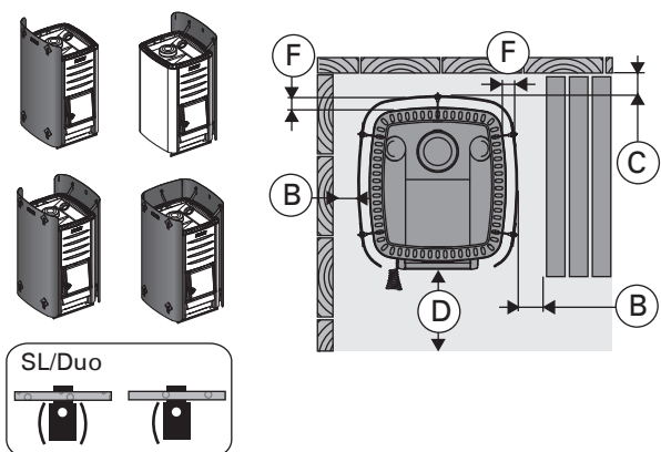
Рисунок 8. Безопасные расстояния с защитными ограждениями (все размеры приведены в миллиметрах) Joonis 8. Ohutuskaugus koos kaitseseinaga (kõik mõõtmised millimeetrites)
