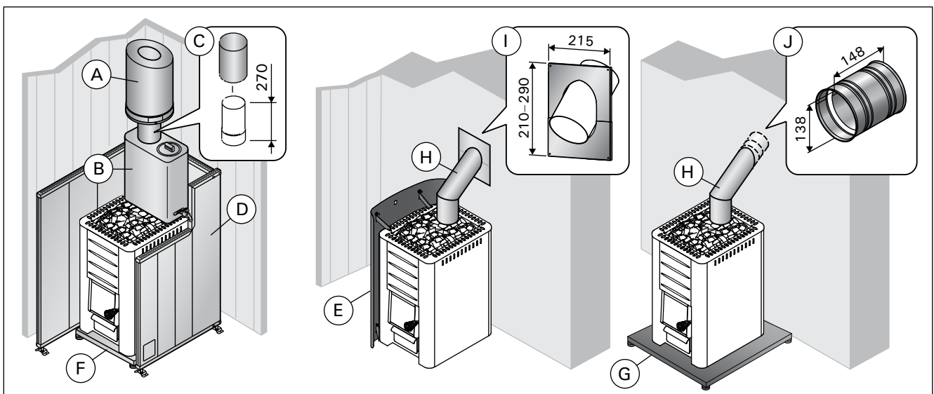
Kuva 13. Lisätarvikkeet (mitat millimetreinä) Bild 13. Tilläggsutrustning (måttene i millimeter)
