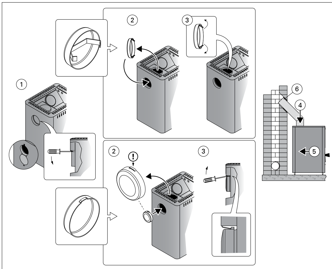
Kuva 10. Kiukaan liittäminen murattuun savuhormiin yläliitântäaukon kautta (mitat millimetreinä)
