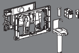
Geberit DuoFresh -moduuli manuaalikytkimelle, sis. raikastinpuikkokehyksen
