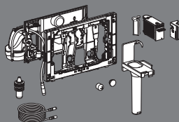
Geberit DuoFresh -moduuli käyttäjäilmaisimella, sis. raikastinpuikkokehyksen
