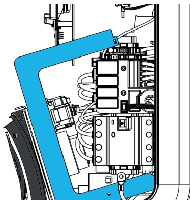
Image 5: Detachable subframe
