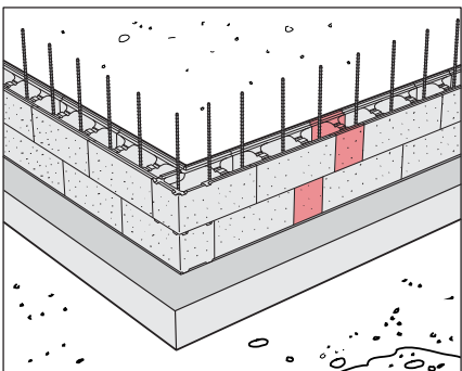
Kuva 11. Sovittepallojen sijoittelu harkkoseinässä.
