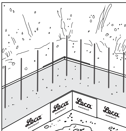
Kuva 7. Esimerkki anturamuotista.
