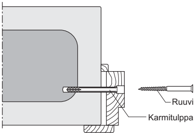
Kuva 15. Puukarmin kiinnityisperiaate kulmaharkkoon.
