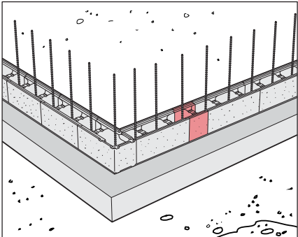
Kuva 12. Harkkoseinän raudoitusperiaate.
