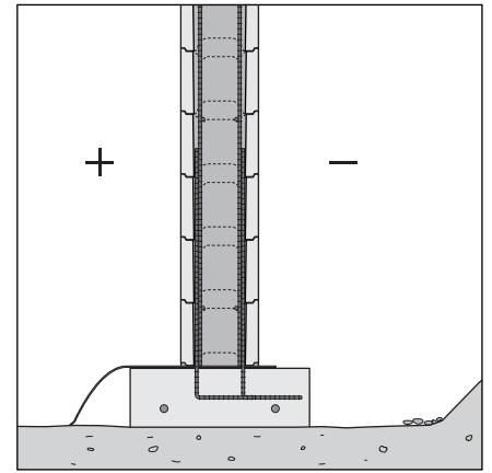
Kuva 13. Harkkoseinän raudoitusperiaate.
