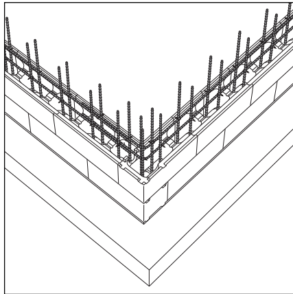
Kuva 12. Harkkoseinän raudoitusperiaate.
