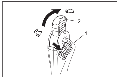
► 1. Apturēšanas slēdžis 2. Akseleratora svira
