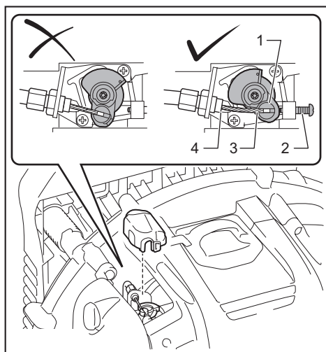
► 1. Gaasiklapp 2. Tühikäigu reguleerimiskruvi 3. Juhttross 4. Gaasiklapi stopper
