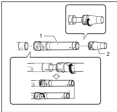
► 1. Длинная/короткая труба 2. Насадка воздухоудовки
