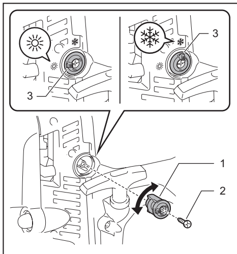
► 1. Jäätumisvastane hoob 2. Kruvi 3. Nupp
