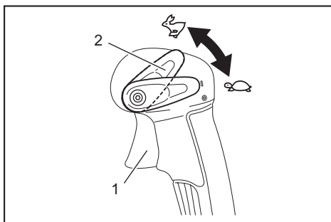
► 1. Kaasuliipaisin 2. Ohjausvivun pysäytin
