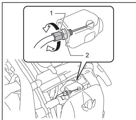
► 1. Trossi reguleerimispolst 2. Kinnitusmutter
