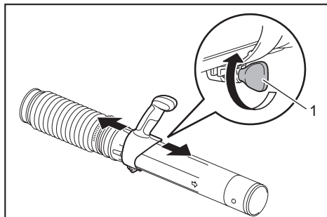
► 1. Spīlējuma skrūve
