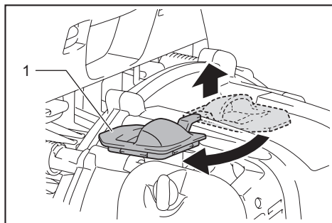
► 1. Plug cover
