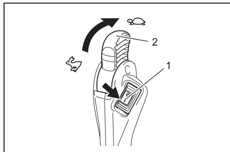
► 1. Pysäytyskytkin 2. Kaasuvipu
