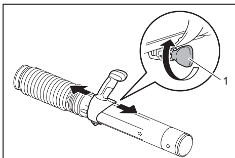
► 1. Klemmeskrue
