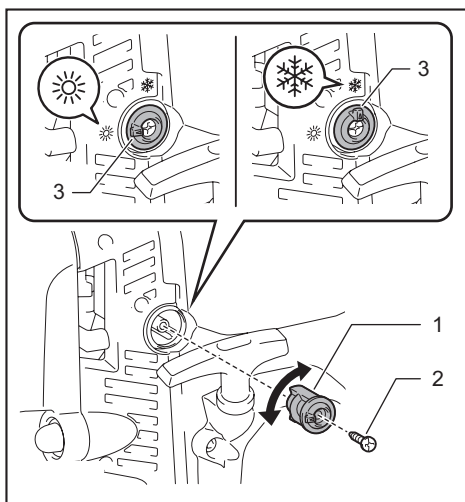
► 1. Antiisingshåndtak 2. Skruer 3. Knott
