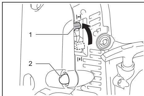
► 1. Chokeyknapp 2. Primerpump
