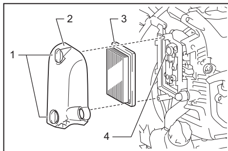
► 1. Rankenėlės varžtai 2. Oro filtro dangtelis 3. Elementas 4. Alsuklis
