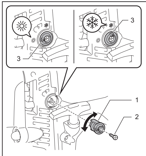
► 1. Pretaizsalšanas svira 2. Skrūve 3. Izcilnis
