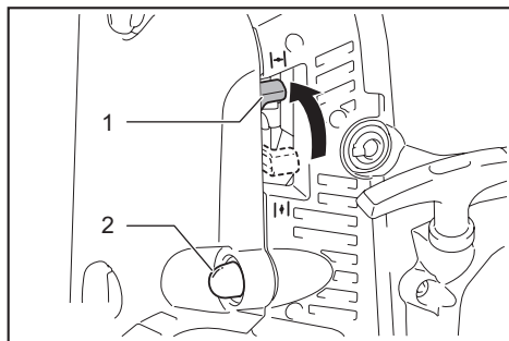
► 1. Õhuklapi hoob 2. Täitepump
