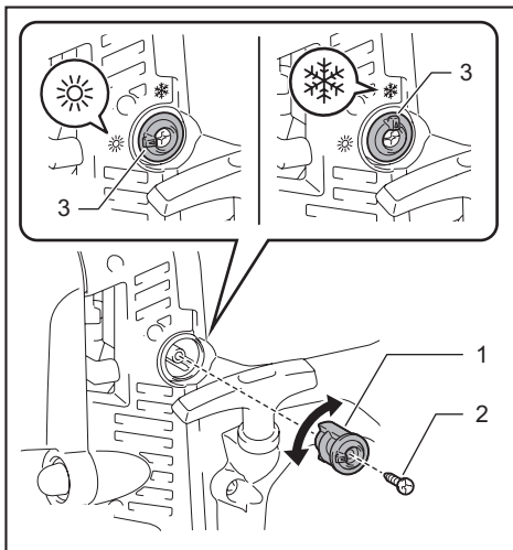
► 1. Anti-isbildningsratt 2. Skruv 3. Markering
