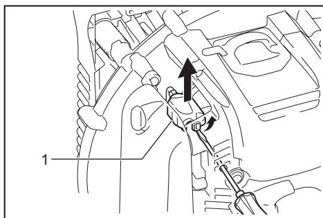
► 1. Karbiuratoriaus dangtelis
