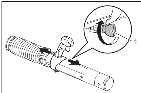
► 1. Spännskruv
