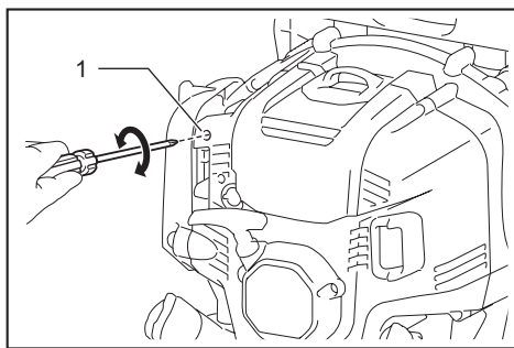
► 1. Joutokäynnin säätöruuvi
