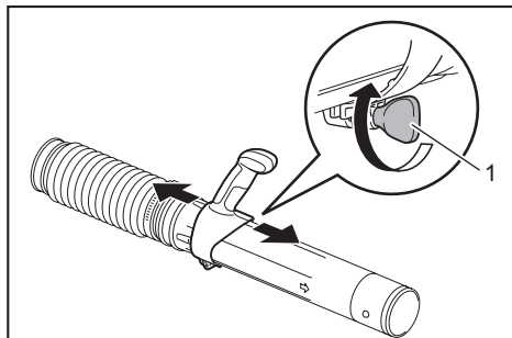
► 1. Spaustuvo sraigtas
