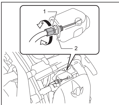
► 1. Kaapelin säätöpultti 2. Kiinnitysmutteri
