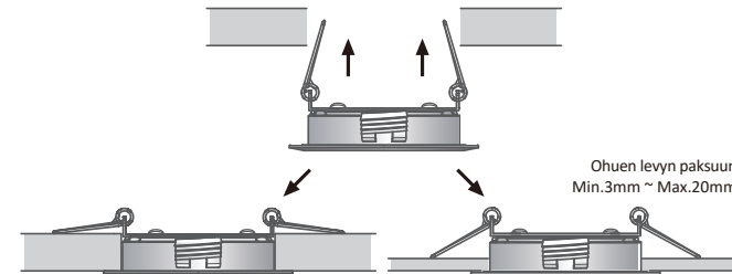
Kuva. 6 Asennus jousikiinnikkeillä
