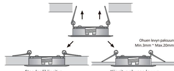
Kuva. 6 Asennus jousikiinnikkeillä
