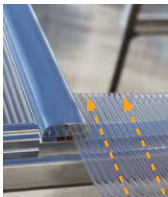
Paneelien liukuasennus
