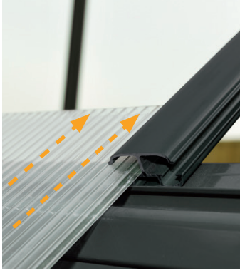
Paneelien liukuasennus
