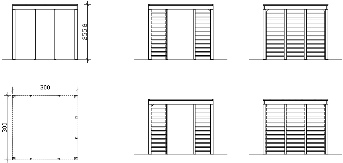
Pohja-, leikkaus- ja julkisivupiirustukset suhteessa 1:100
