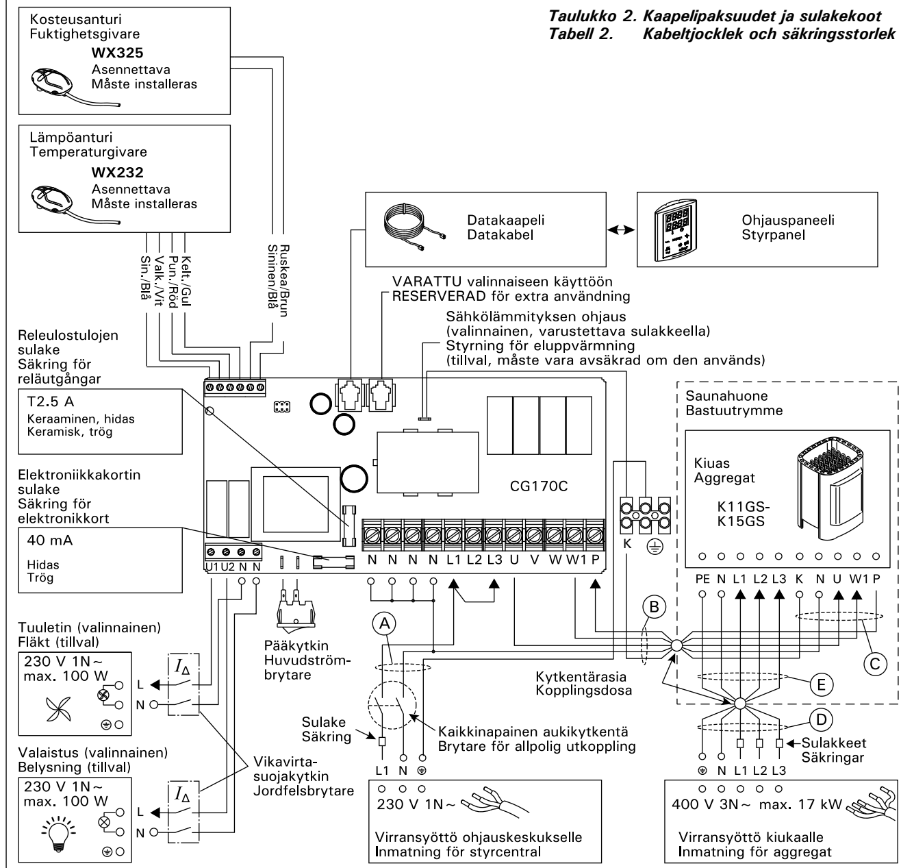
Kuva 6. Sähkökytkennät (K11GS–K15GS) Bild 6. Elektriska anslutningar (K11GS–K15GS)
