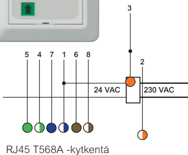
RJ45 T568A -kytkentä
