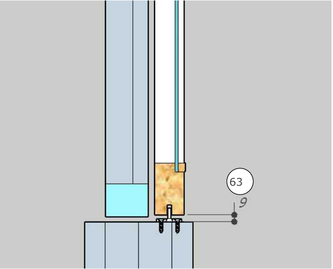
Hav 4+3 liukuovi väliseinässä Lo-1
