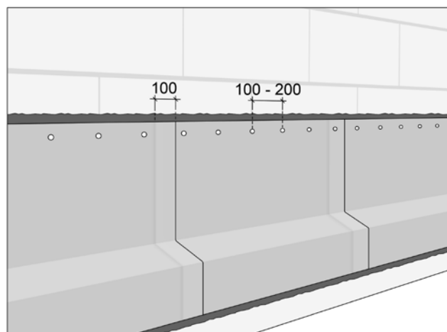
Mekaaninen kiinnitys ja saumojen limitykset.
