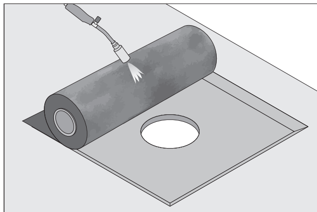
Laippapolar kermiä asennus kaivon pohjalle.
