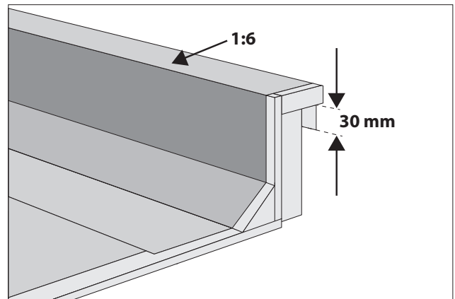
Räystään tulvakermi.
