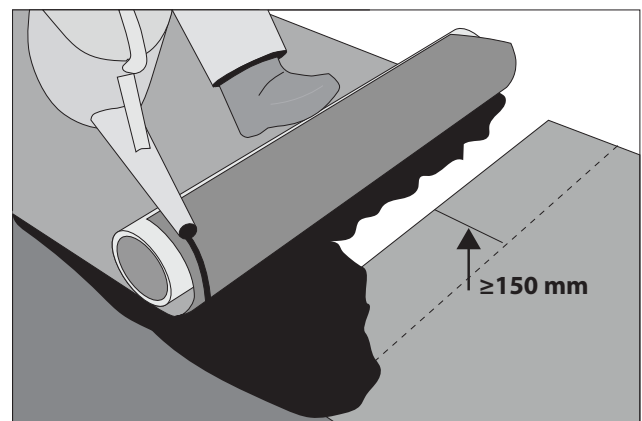
Liimaus, sivu- ja päätysaumojen limitykset.
