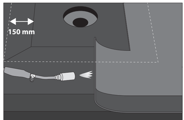
Pintakermin liittäminen kaivon.
