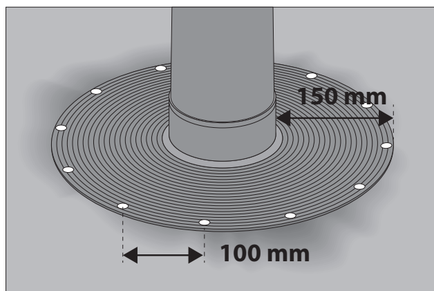
Alipainetuulettimen asennus.
