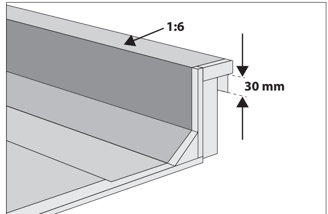
Räystään tulvakermi.
