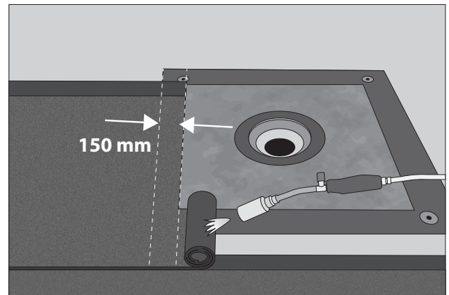
Aluskermi liittäminen kaivon.
