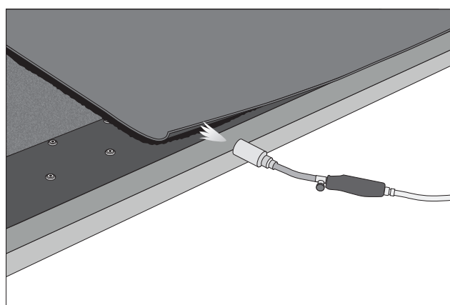
Pintakermin liittäminen tippapeltiin.
