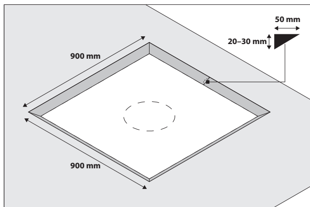
Kaivopesä
