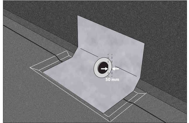
Aluskermi- n liitäntä ulosheittäjään.
