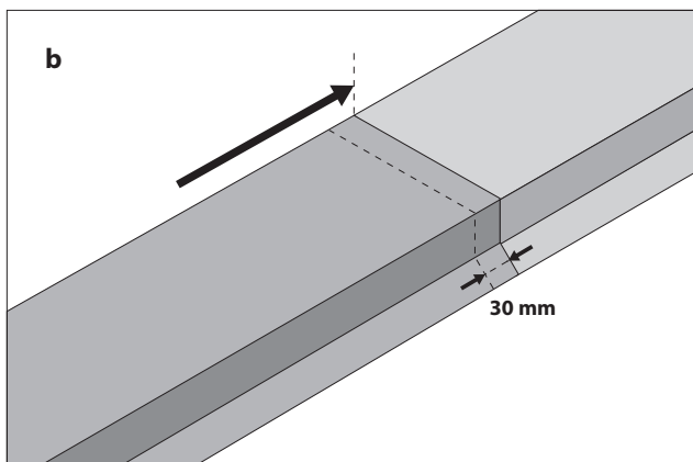
Tippapellin jatkaminen.
