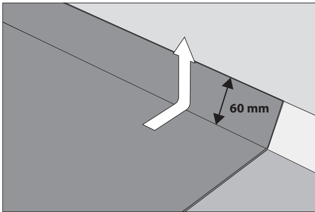
Vaakapinnan kermiä liitos holkkarimaan.
