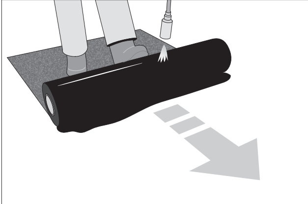
Kauttaaltaan hitsaaminen.
