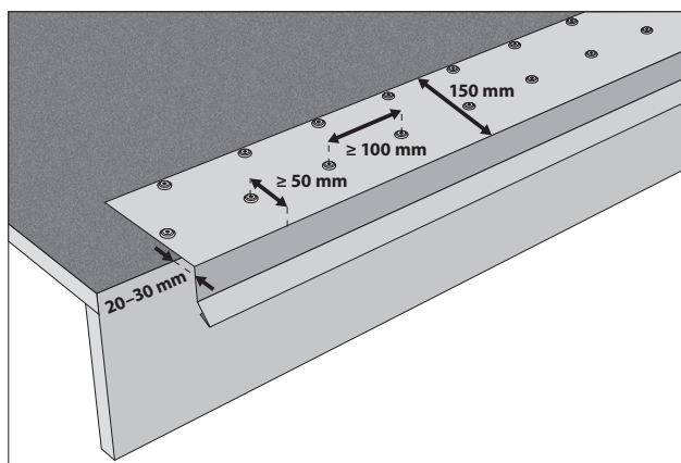
Tippapellin kiinnittäminen.
