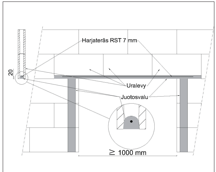
Kuva 7.2 aukonylytys uralevyllä
