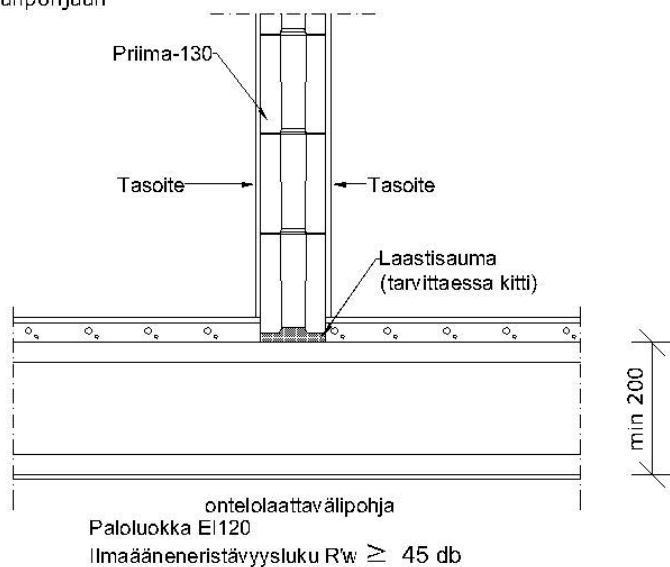
DET 1. Alapään liitos ontelolaatta välipohjaan
