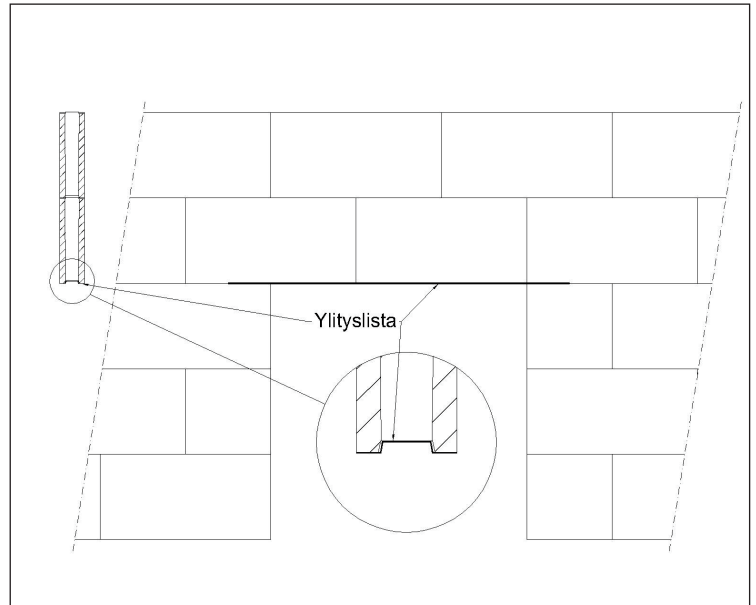
Kuva 7. HB-Priima 88 aukonylytys aukonylytyslistalla
