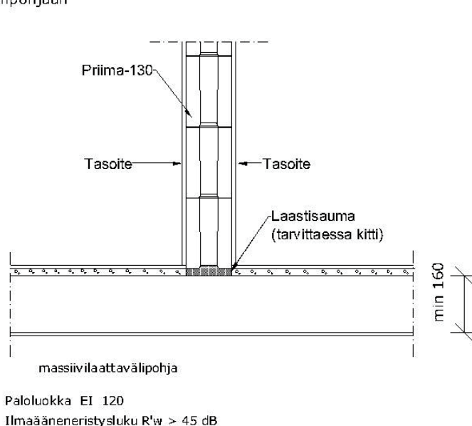
DET 2. Alapään liitos massiivilaatta välipohjaan
