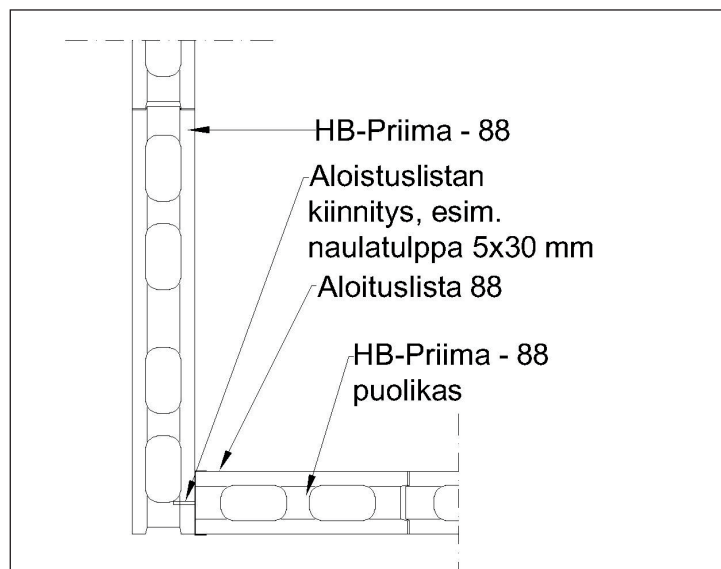
Kuva 6.1 Priima-88 kulma kourualoituslistalla
