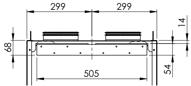
Seinäasennustelineen mitat
