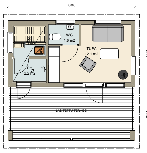
tupaa, sauna, wc
