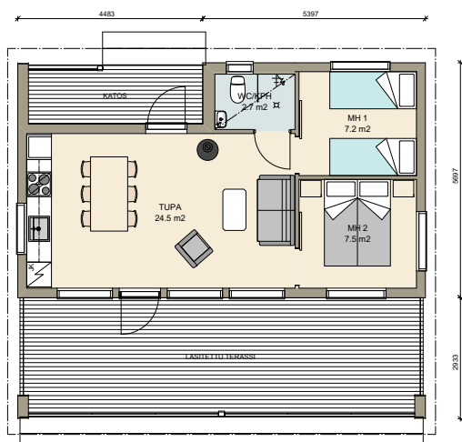
tupa, 2 mh, wc
