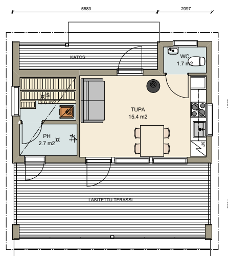
tupaa, sauna, wc
