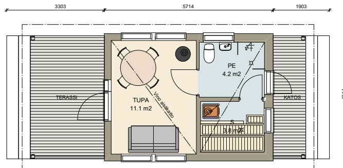
tupa, sauna, wc
