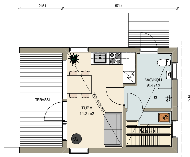
tupaa, sauna, wc
