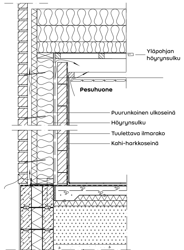
Puurunkoinen ulkoseinä, jonka sisäpuolelle on tehty verhomuuraus
