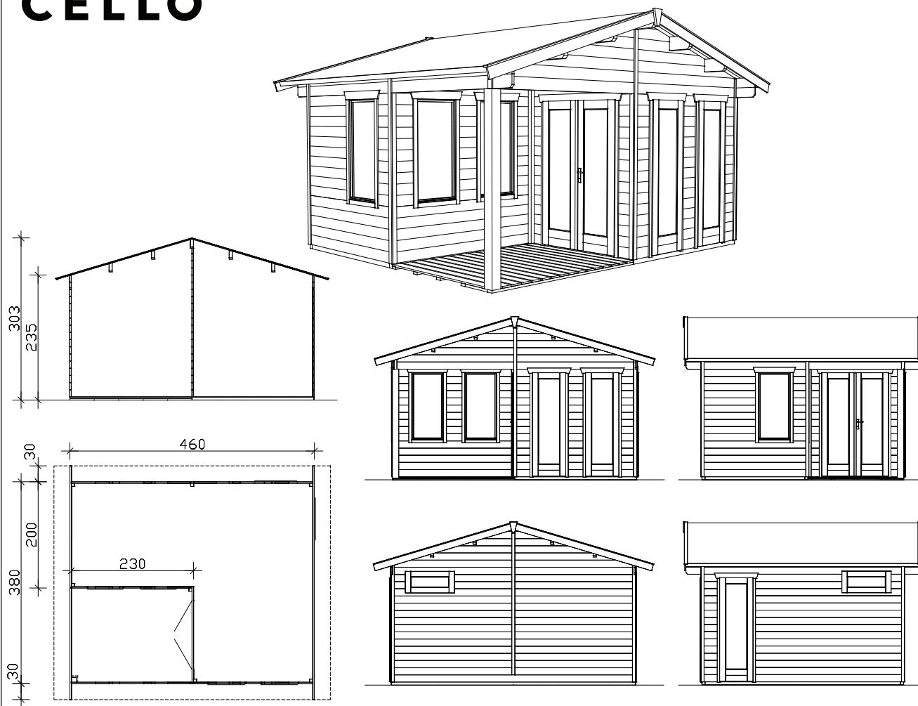
Põhiplaan, lõige ja vaated M 1 :100
