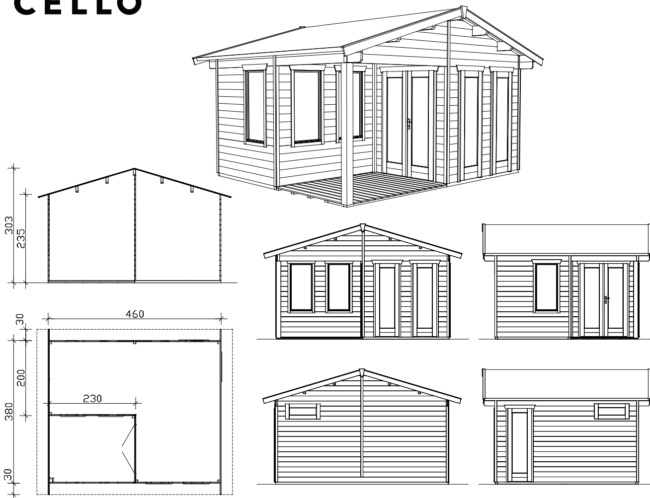
Ritning, snitt och bilder M 1 :100
