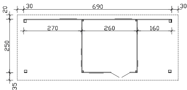
Põhiplaan, lõige ja vaated M 1 :100
