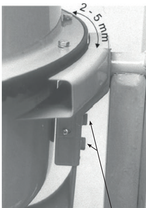
M10x25
