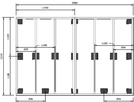
Pohjan mitat ja perustuskuv
