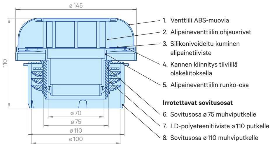
Merika®-alipaineventtiili 70/75/100/110
