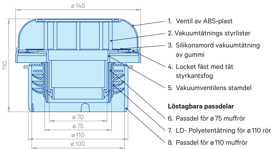
Merika-vakuumventilens 70/75/100/110 konstruktion
