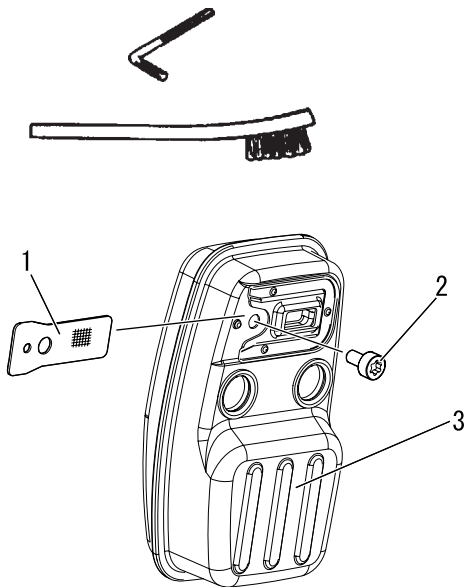
1. Gnistfångarskärm
