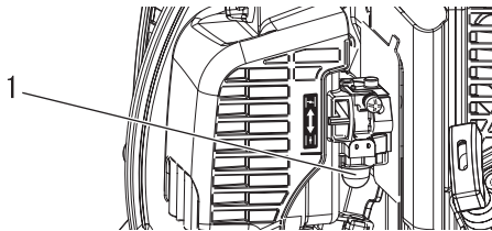
1. Gasspjällets spak
