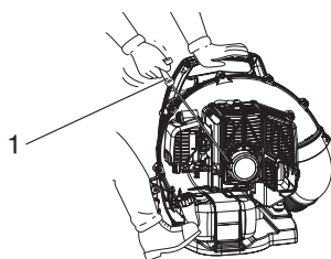
1. Startrepanordningens handtag
