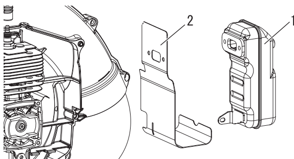
1. Ljuddämpare
