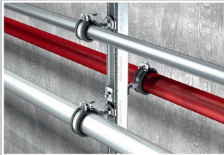
FHS Clix pikakiinnityspala kierretapilla
