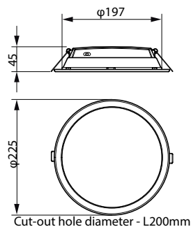
DN065B G3 LDNR LED20/CCT 19.5W D200 RD
