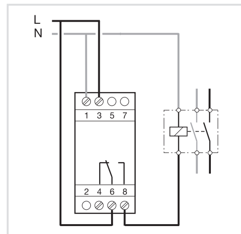
Bilde 2: koblingsskjema EGN103 (1 utgang)
