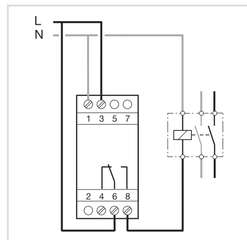
Bild 2: kopplingsschema EGN103 (1 utgång)
