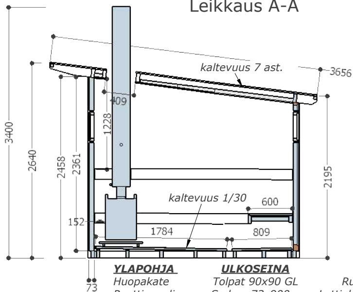
Leikkaus A-A
