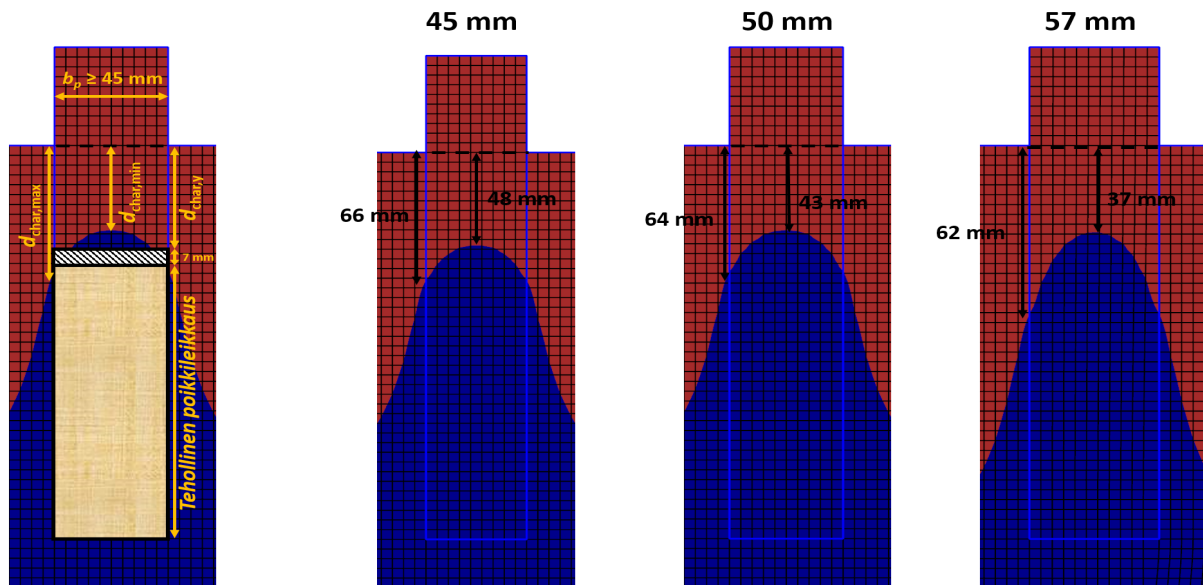
Kuva 1. Tehollisen poikkileikkauksen määrittäminen (vasemmalla) ja puupalkin hiiltymissyvyys lasketuissa tapauksissa, kun sen sivuja suojaa Kooltherm®-eriste.
