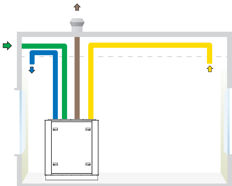
CASA R15 kanavaliitännät.
