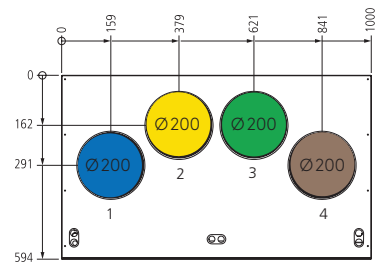
CASA W9 R, oikeakätinen versio
