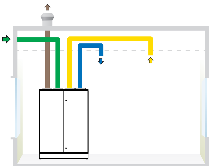
W9 L kanavaliitännät.
