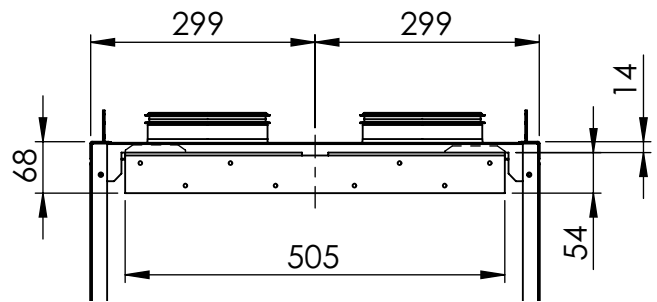
Seinäasennustelineen mitat
