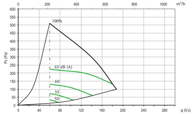
Äänitehotaso ulkoilmakanavaan
