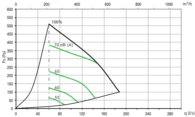
Äänitehotaso tuloilmakanavaan
