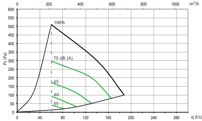
Äänitehotaso ulospuhallusilmakanavaan
