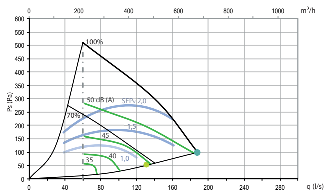
Ilmamäärät ja äänitehotaso ympäristöön
