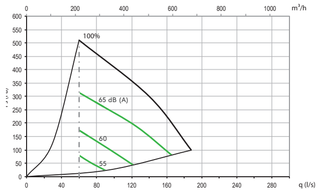
Äänitehotaso poistoilmakanavaan
