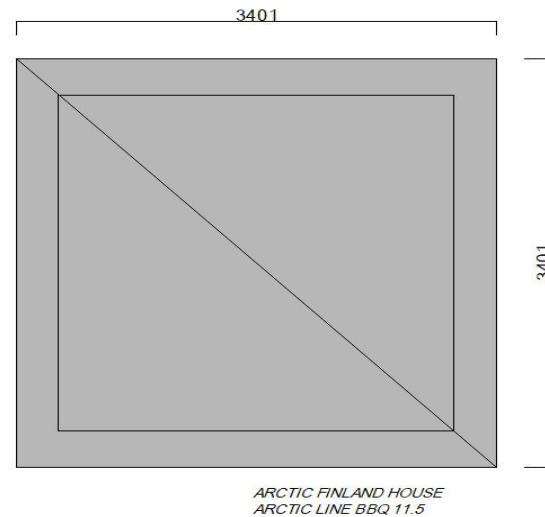
Perustukset pohjakuva
