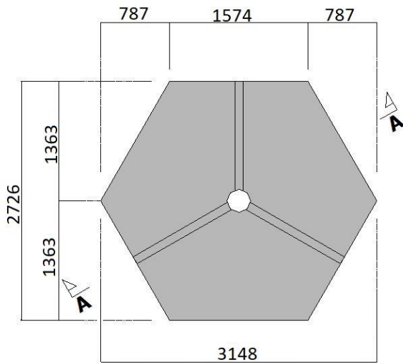
Perustukset pohjakuva
