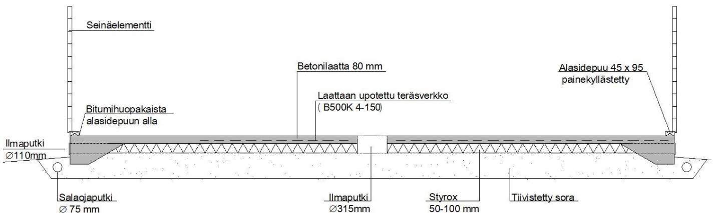
Perustukset Leikkaus A - A:
